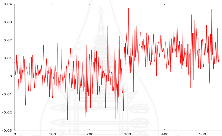
ภาพที่ 4.1 กราฟแสดงข้อมูลอัตราผลตอบแทนรายวันของกองทุนเปิด BCAP SET100 ETF จำนวน 544 วัน หรือตั้งแต่ เดือนกันยายน 2560 ถึงเดือน ธันวาคม 2562
