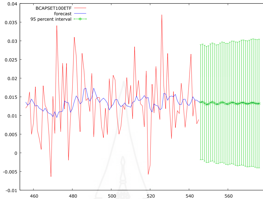
ภาพที่ 4.4 กราฟ แสดงการพยากรณ์อัตราผลตอบแทนเฉลี่ยของกองทุนเปิด BCAP SET100 ETF
