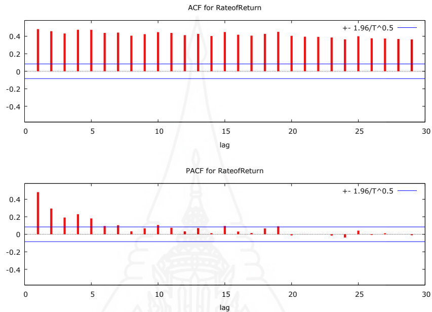
ภาพที่ 4.2 กราฟ ACF และ PACF ของอัตราผลตอบแทนรายวันกองทุนเปิด BCAP SET100 ETF
