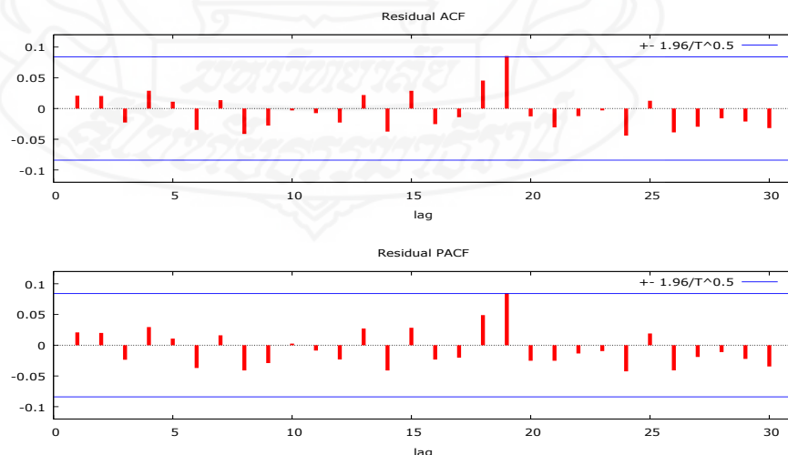
ภาพที่ 4.3 กราฟ Correlogram ของข้อมูลเมื่อหาผลต่างครั้งที่ 1 แล้ว
